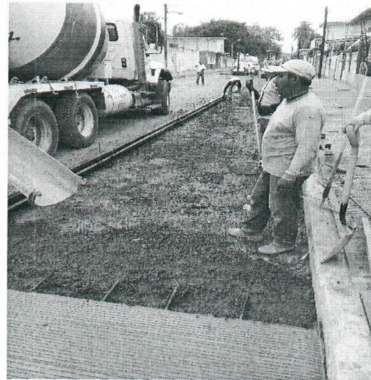
SUMINISTRO Y TENDIDO DE CONCRETO HIDRAULICO
