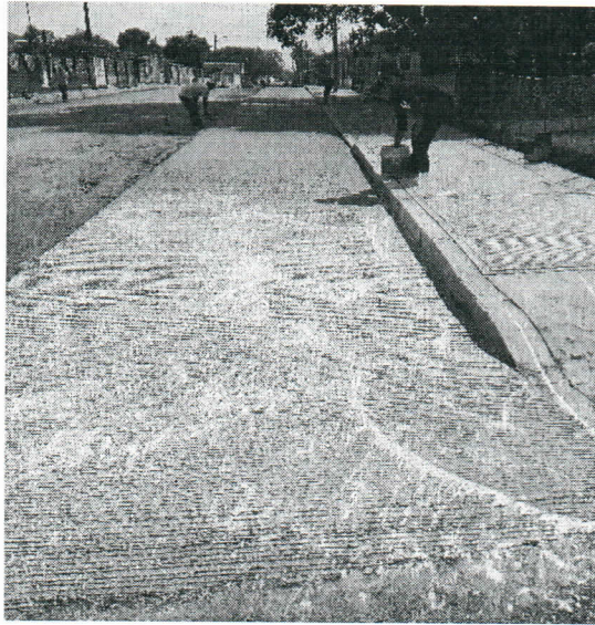
SUMINISTRO Y APLICACIÓN DE CURACRETO
